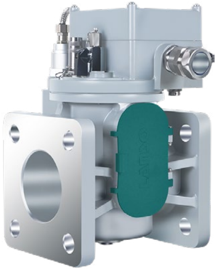
TR-80R 智能型气体继电器
