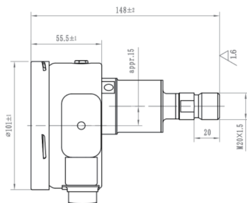
轴向尺寸图
