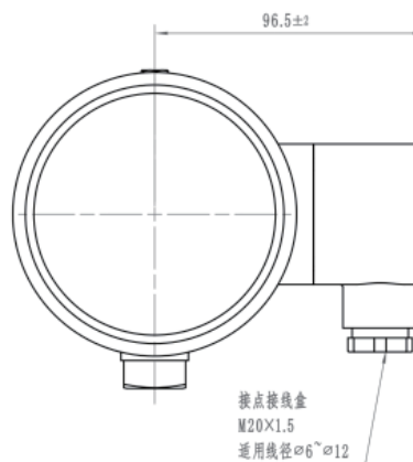
轴向尺寸图
