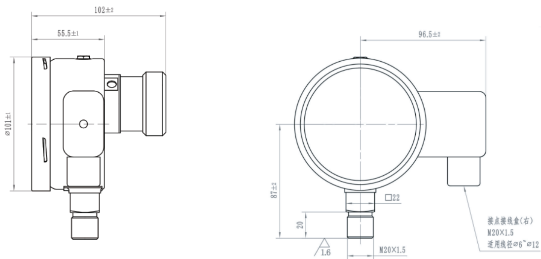
径向6点尺寸图
