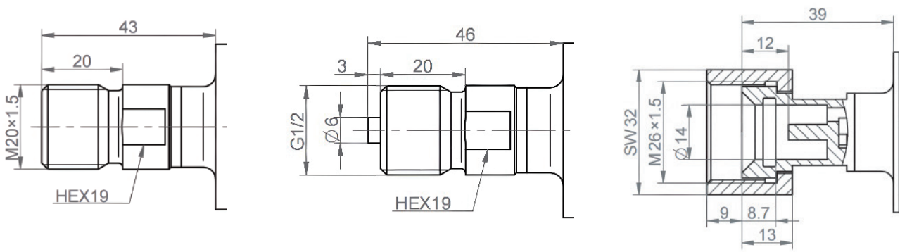
选项1 M20*1.5
