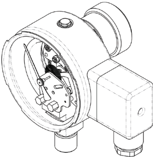
3组接点
