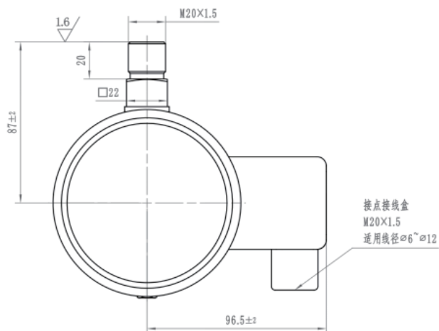
径向12点尺寸图
