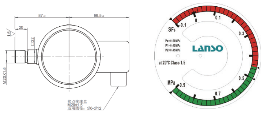
侧装度盘 (9点钟)
