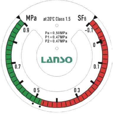
倒装度盘
