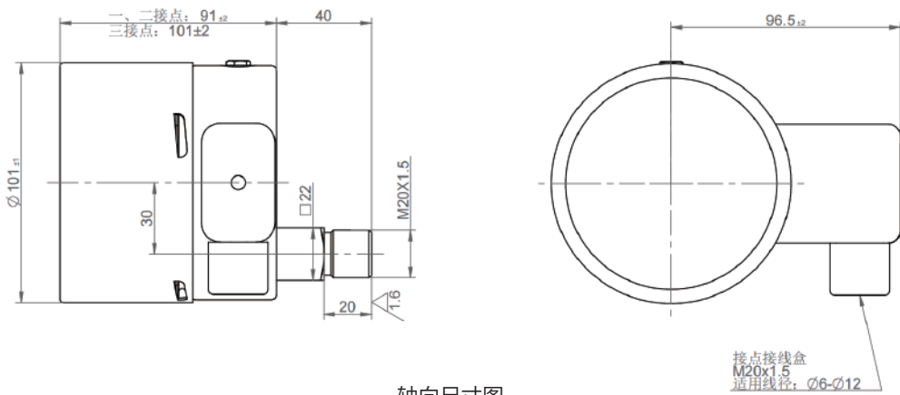
轴向尺寸图
