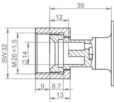
选项3 M26*1.5
