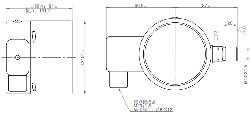
径向3点尺寸图
