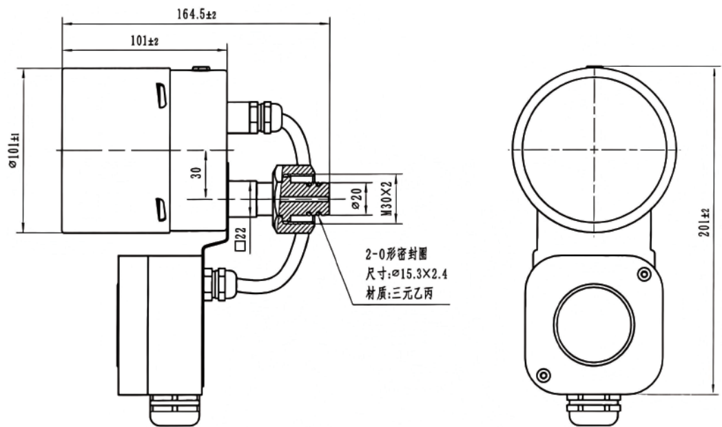
ZMJ100P 独立接线盒款
