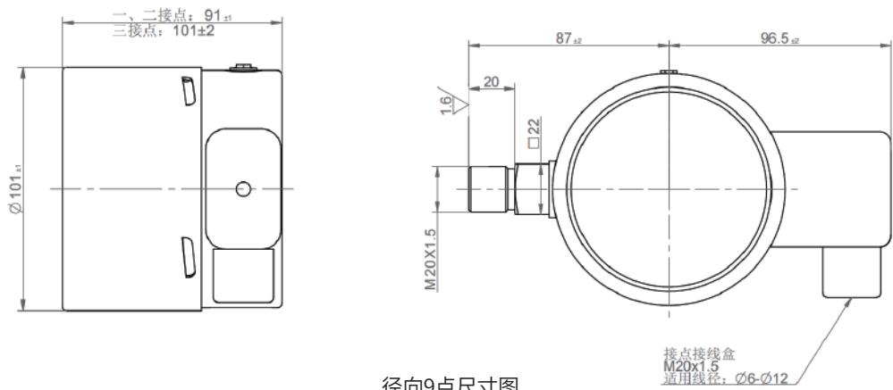
径向9点尺寸图
