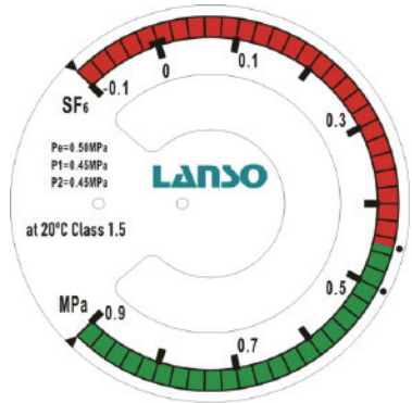
侧装度盘 (9点钟)
