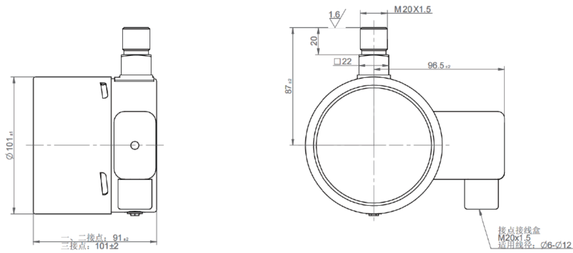
径向12点尺寸图
