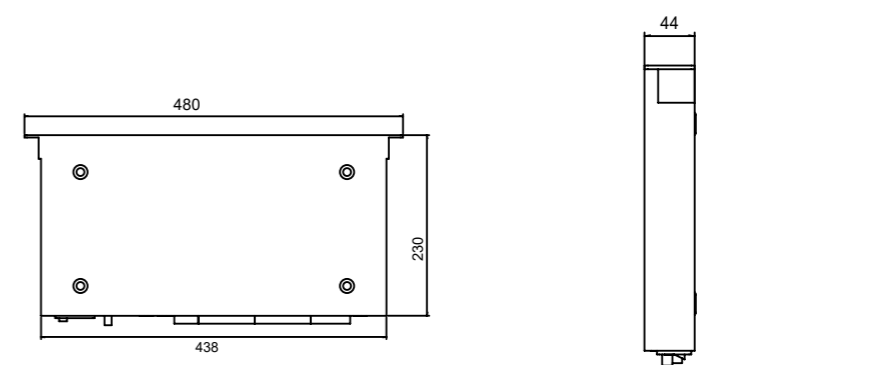
IED-8240 外形图
